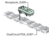
Receptacle — 15 Amp
